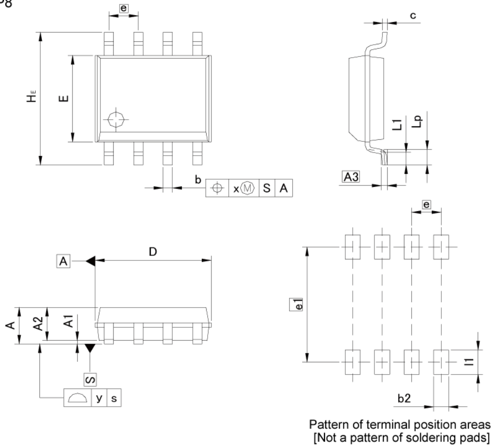
SOP8
