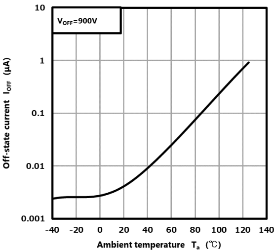
Fig. 12.7 I_{OFF} - T_a
