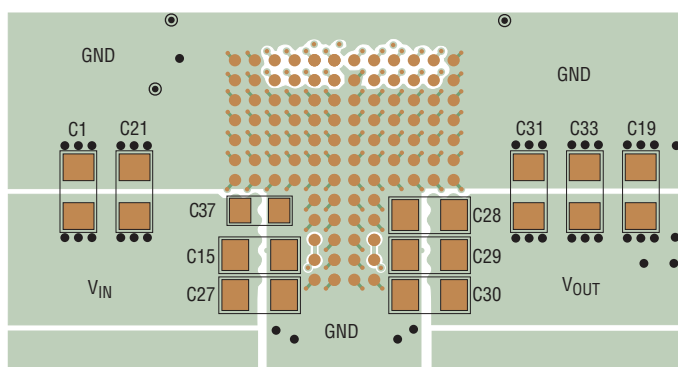
(b) LTM4712 Bottom Layer
