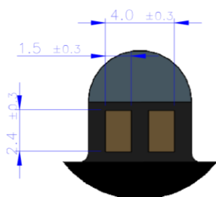
細部放大圖 A 縮放 4 : 1
