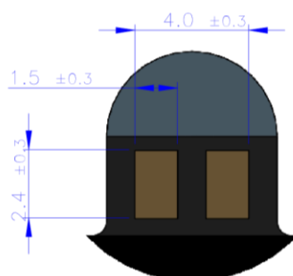
細部放大圖 A 縮放 5 : 1
