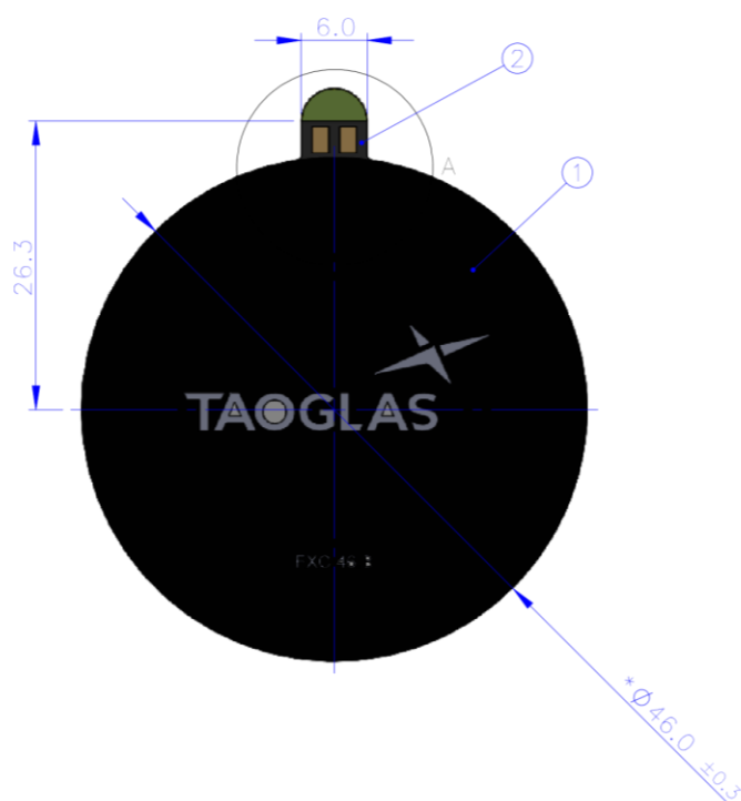
細部放大圖 A 縮放 2 : 1
