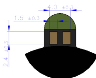
細部放大圖 A 縮放 3 : 1
