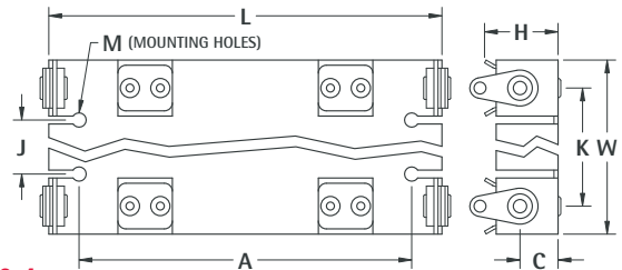
DWG. 4
