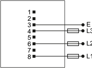
3P3W
