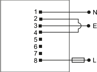
1P2W + E
