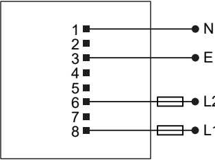
1P3W
