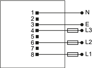
3P4W
