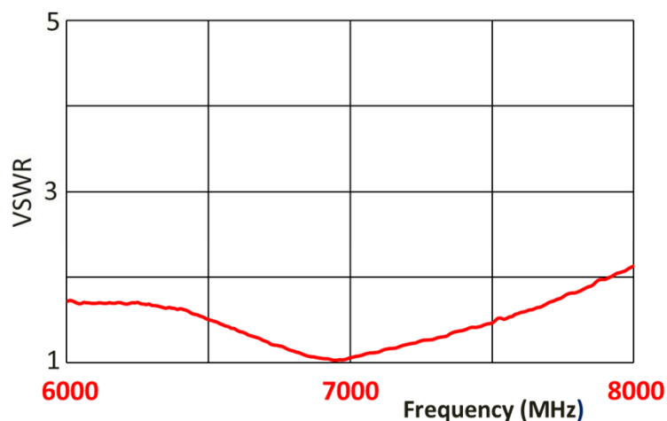
VSWR
