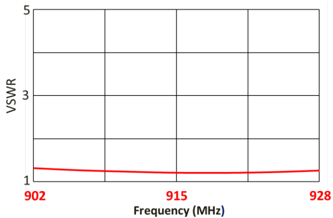
VSWR
