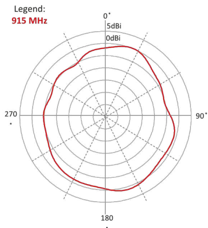
Elevation 1
