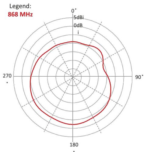
Elevation 1
