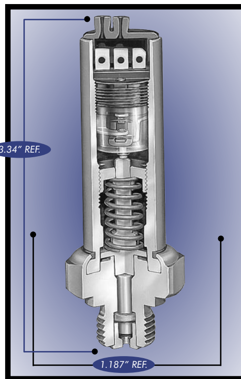
Piston Type
