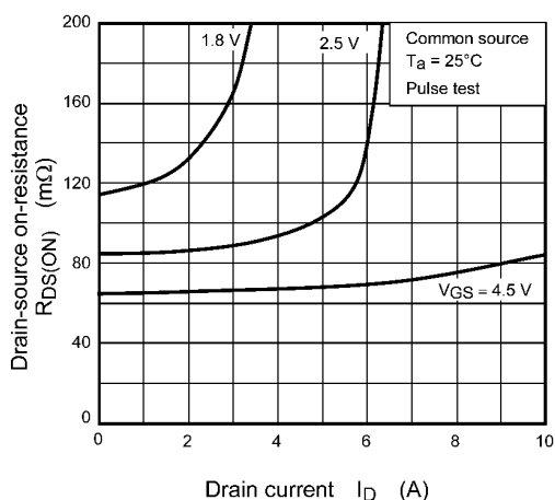
Fig. 8.5 R_{DS(ON)} - I_D
