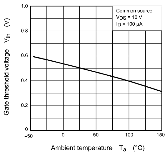
Fig. 7.7 V_{th} - T_a
