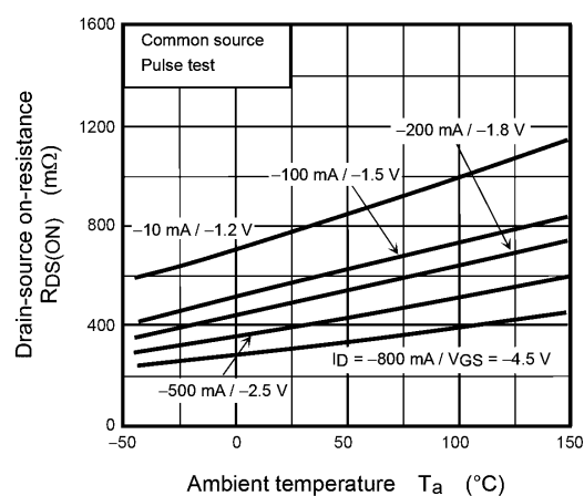
Fig. 7.2.5 R_{DS(ON)} - T_a
