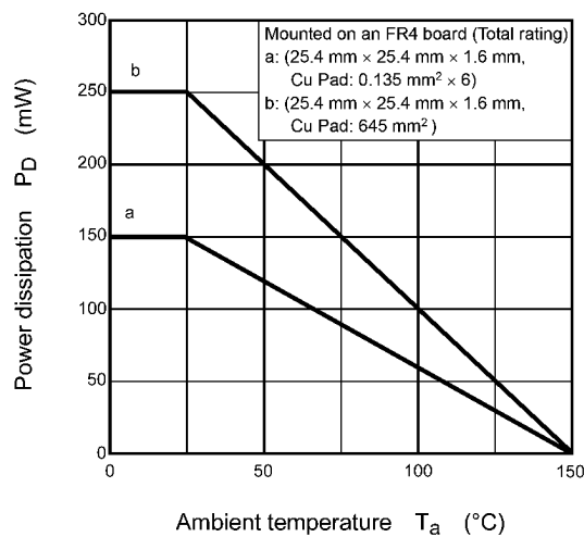
Fig. 7.3.1 P_D - T_a
