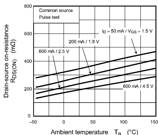
Fig. 7.1.5 R_{DS(ON)} - T_a
