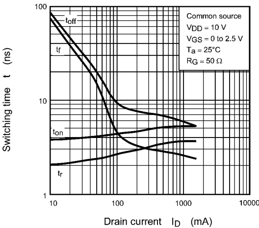
Fig. 7.1.10 t - I_D
