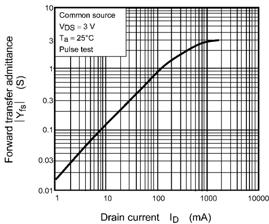
Fig. 7.1.7 |Y_{fs}| - I_D
