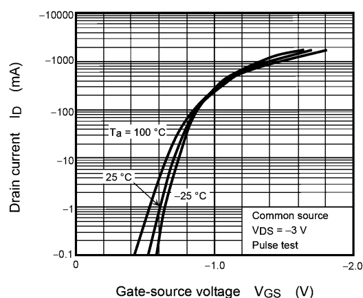
Fig. 7.2.2 I_D - V_{GS}
