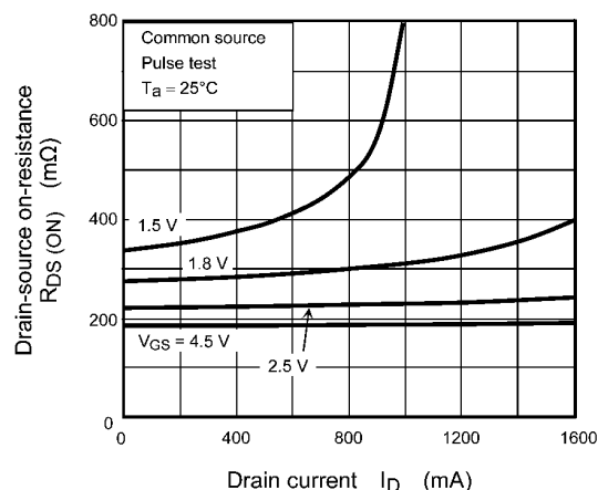
Fig. 7.1.4 R_{DS(ON)} - I_D
