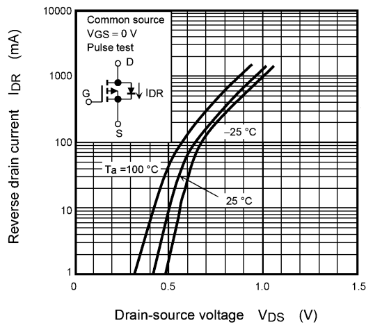
Fig. 7.2.9 I_{DR} - V_{DS}
