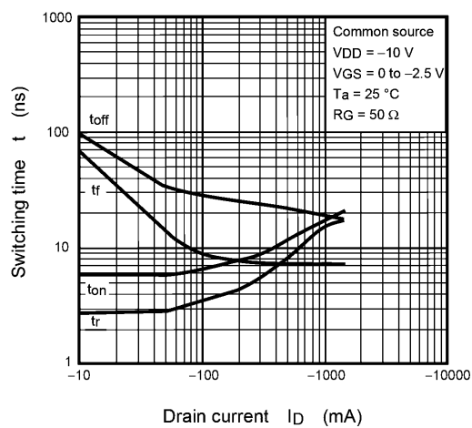
Fig. 7.2.11 t - I_D
