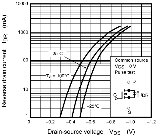
Fig. 7.1.8 I_{DR} - V_{DS}
