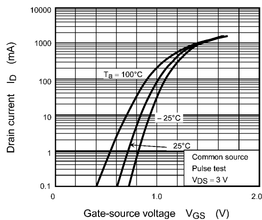
Fig. 7.1.2 I_D - V_{GS}
