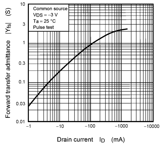
Fig. 7.2.8 |Y_{fs}| - I_D
