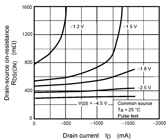
Fig. 7.2.6 R_{DS(ON)} - I_D
