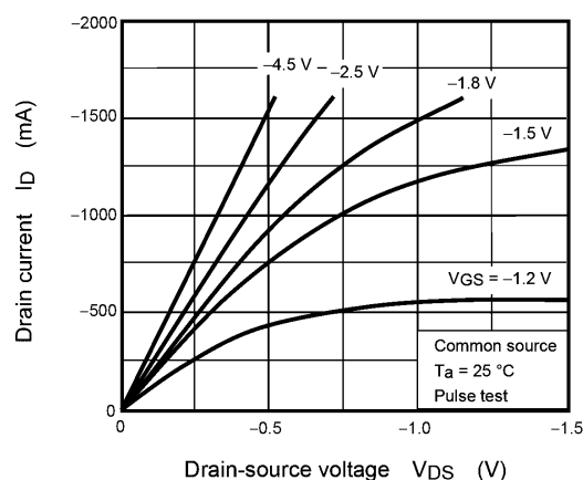
Fig. 7.2.1 I_D - V_{DS}
