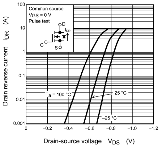
Fig. 8.9 I_{DR} - V_{DS}
