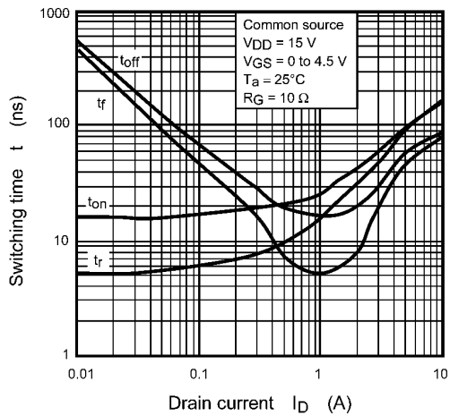
Fig. 8.11 t - I_D
