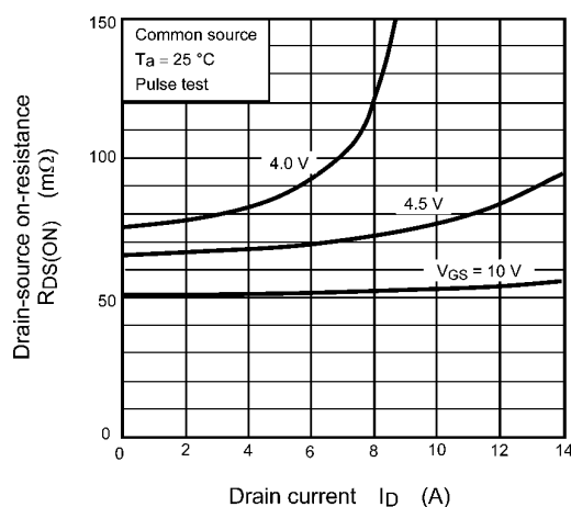
Fig. 8.2 R_{DS(ON)} - I_D
