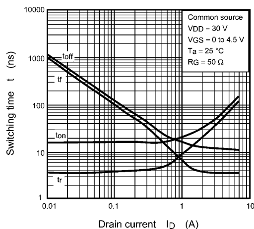
Fig. 8.4 t - I_D
