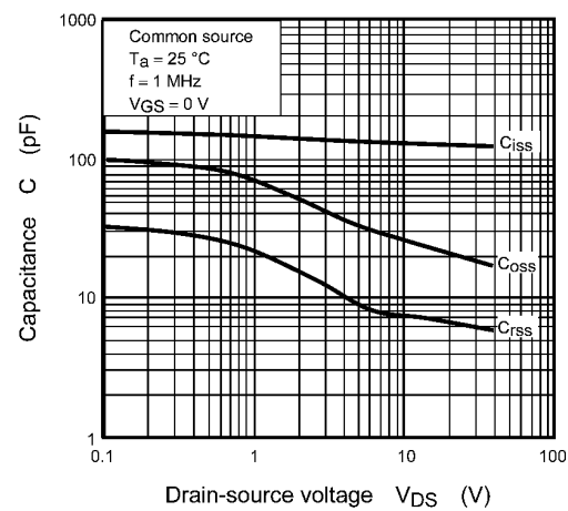
Fig. 7.10 C - V_{DS}
