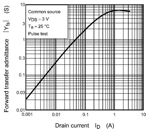
Fig. 7.8 |Y_{fs}| - I_D
