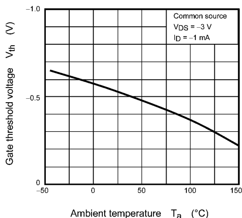
Fig. 7.6 V_{th} - T_a
