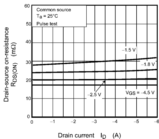
Fig. 7.4 R_{DS(ON)} - I_D
