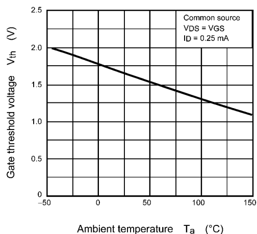
Fig. 7.6 V_{th} - T_a
