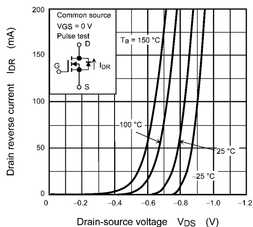
Fig. 7.8 I_{DR} - V_{DS}
