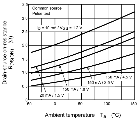
Fig. 7.6 R_{DS(ON)} - T_a
