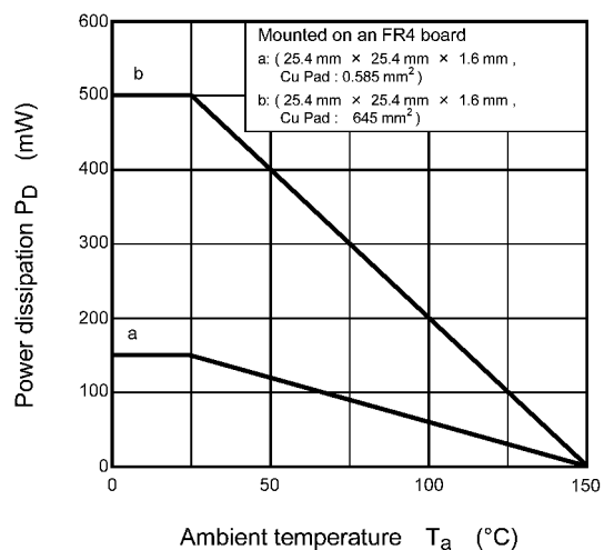
Fig. 7.13 P_D - T_a
