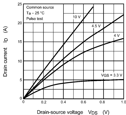
Fig. 8.1 I_D - V_{DS}
