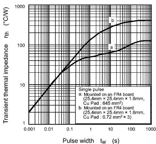
Fig. 8.12 r_{th} - t_w
