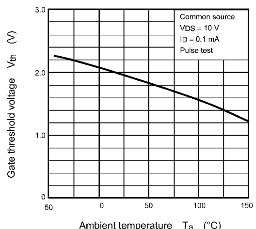
Fig. 8.6 V_{th} - T_a
