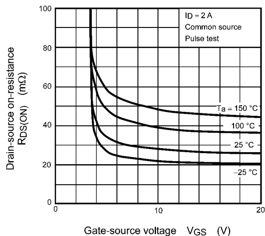
Fig. 8.3 R_{DS(ON)} - V_{GS}
