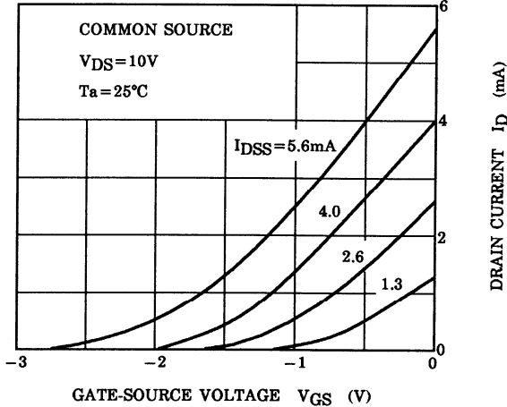
I_D - V_{GS}
