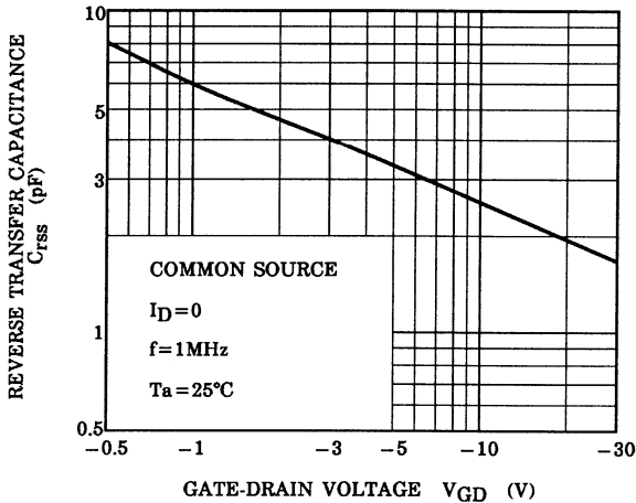
C_{rss} - V_{GD}
