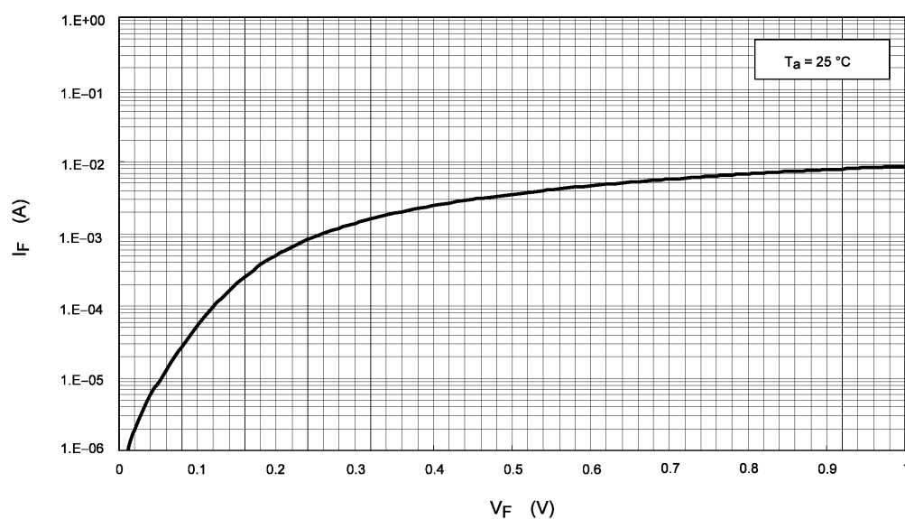
Fig. 9.1 I_F - V_F
