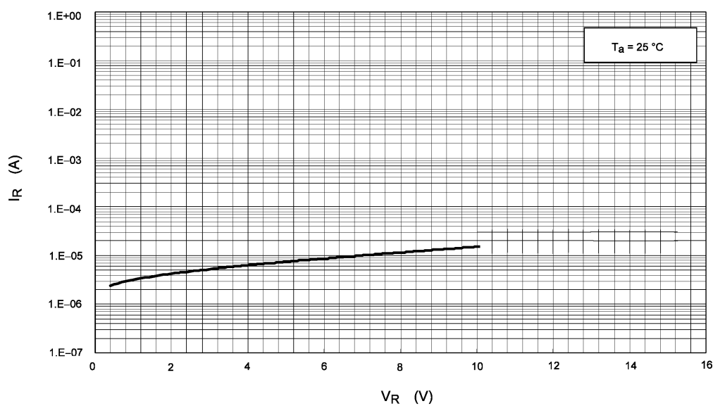
Fig. 9.2 I_R - V_R
