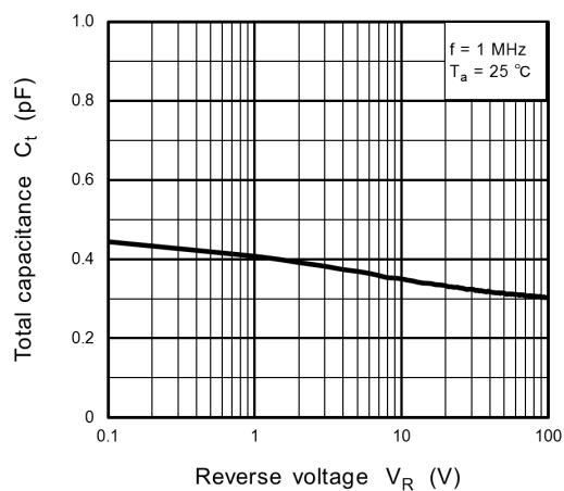
Fig. 7.3 C_t - V_R
