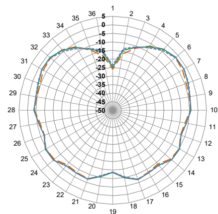
XZ-Plane Gain
