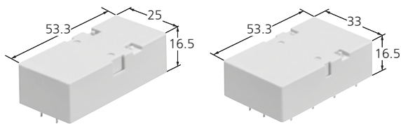
4 poles
