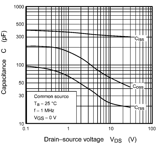
Fig. 8.10 C - V_{DS}
