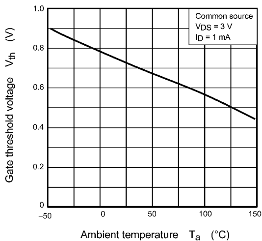
Fig. 8.7 V_{th} - T_a
