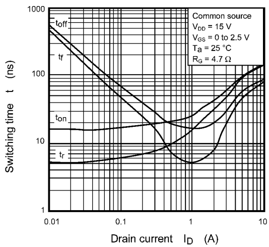
Fig. 8.11 t - I_D
