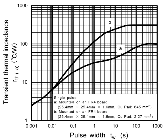
Fig. 8.11 r_{th} - t_w
