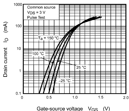
Fig. 7.2 I_D - V_{GS}
