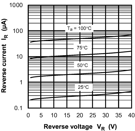
Fig. 9.2 I_R - V_R
