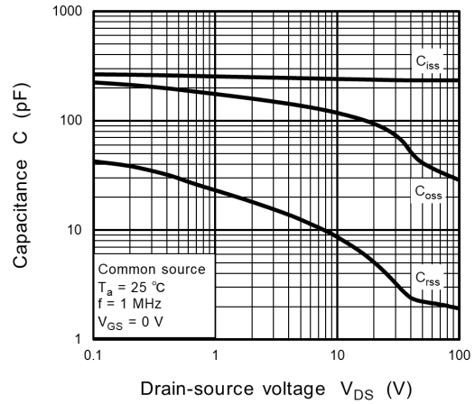
Fig. 8.8 C - V_{DS}
