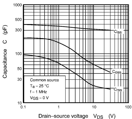
Fig. 8.1.9 C - V_{DS}
