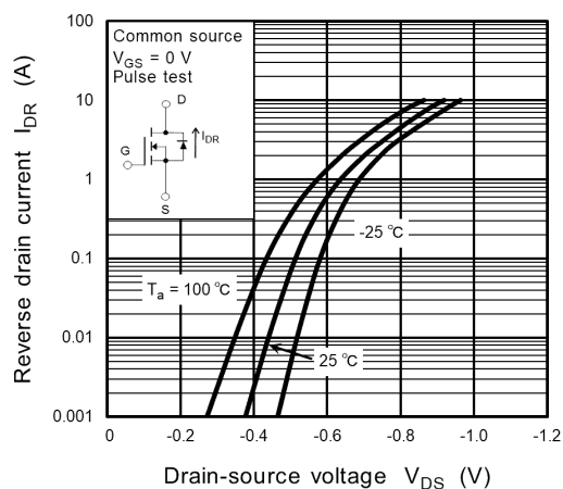
Fig. 8.1.8 I_{DR} - V_{DS}
