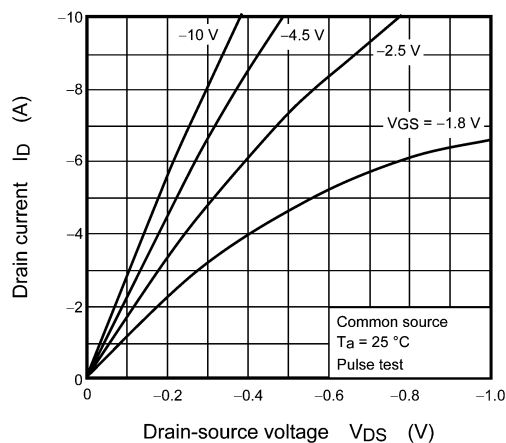
Fig. 8.2.1 I_D - V_{DS}
