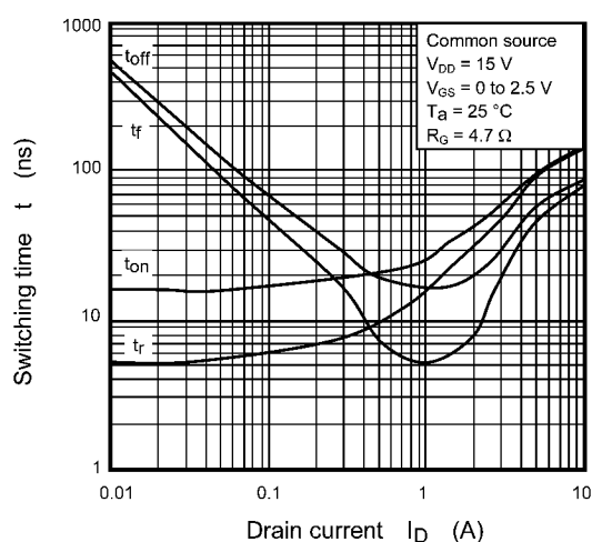
Fig. 8.1.10 t - I_D
