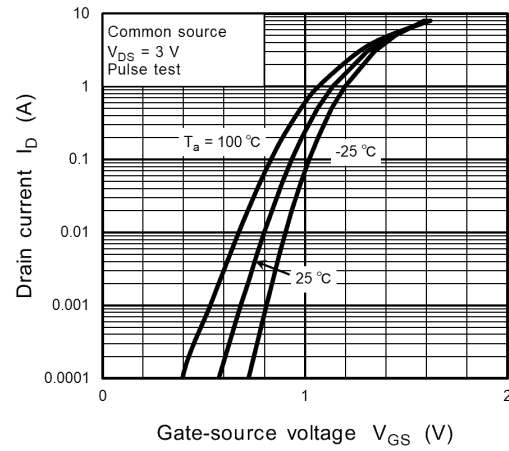
Fig. 8.1.2 I_D - V_{GS}
