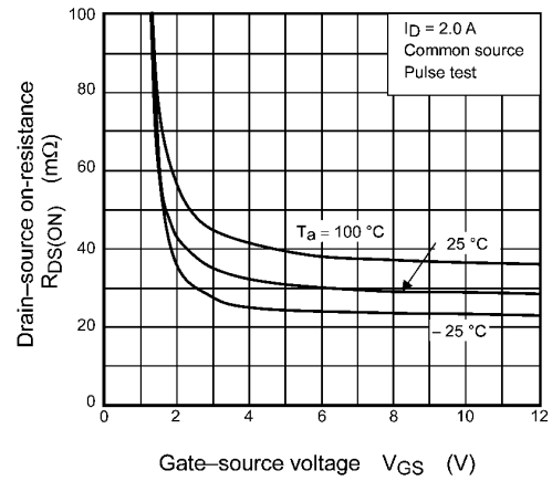
Fig. 8.1.4 R_{DS(ON)} - V_{GS}
