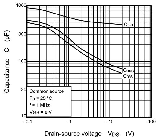
Fig. 8.2.8 C - V_{DS}
