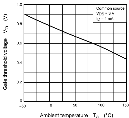
Fig. 8.1.7 V_{th} - T_a
