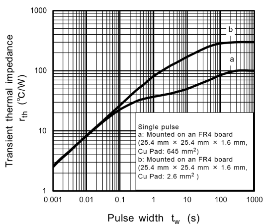
Fig. 8.12 r_{th} - t_w
