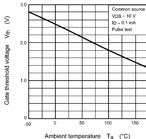
Fig. 8.6 Vth - Ta
