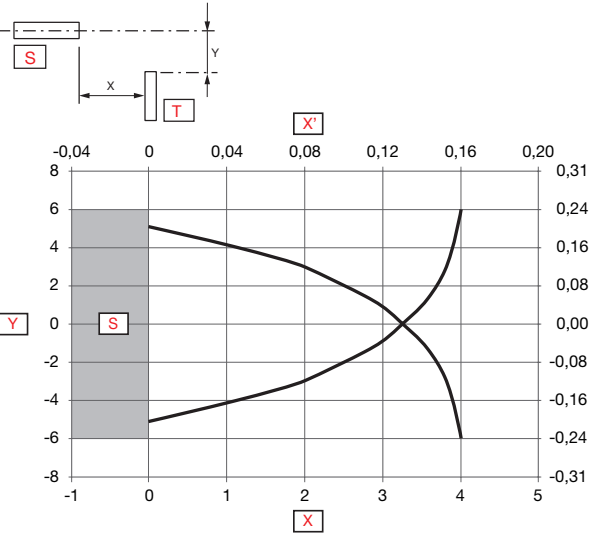
Fig. 4 Flush
