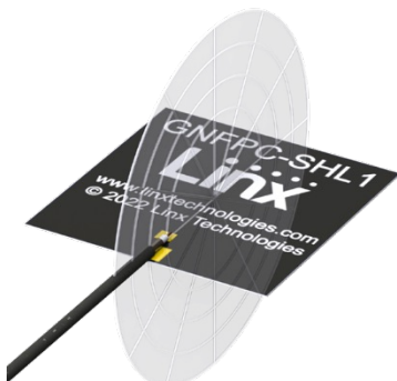
YZ-Plane Gain
