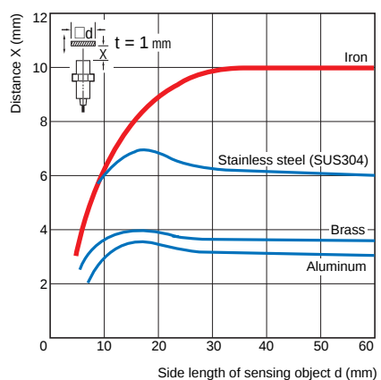
E2E2-X10MC□/I-X10MY□
