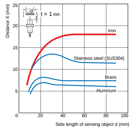
E2E2-X18MC□/I-X18MY□
