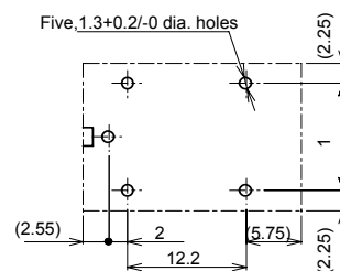
SPDT
