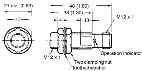
Fig. 16: E2E-X5E□-M1/F□-M1
