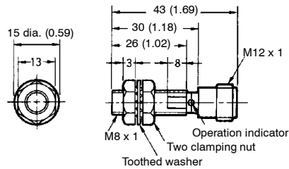
Fig. 14: E2E-X2E□-M1/F□-M1
