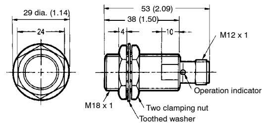
Fig. 16: E2E-X5E□-M1/F□-M1
