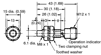
Fig. 13: E2E-X2ME□-M1/F□-M1
