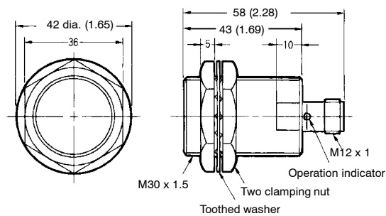
Fig.18: E2E-X10E□-M1/F□-M1
