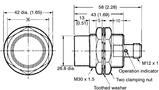
Fig. 19: E2E-X18ME□-M1/F□-M1
