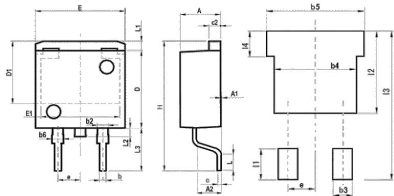
TO-263L, (TO-263L)
