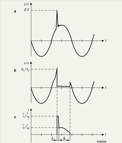
Bild 19a Wechselspannung mit überlagerter Überspannungsspitze
