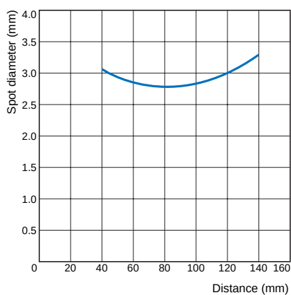
E3Z-L□1(L□6)
