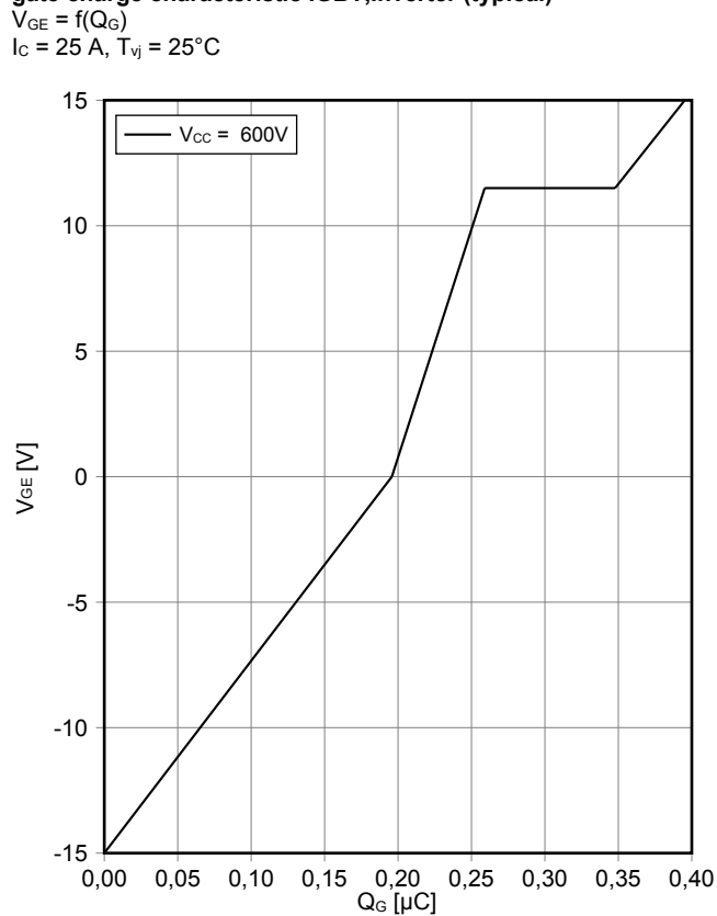
Gateladungs Charakteristik IGBT, Wechselrichter (typisch) gate charge characteristic IGBT, Inverter (typical) V_{GE} = f(Q_G) I_C = 25\text{ A} , T_{vj} = 25^\circ\text{C}
