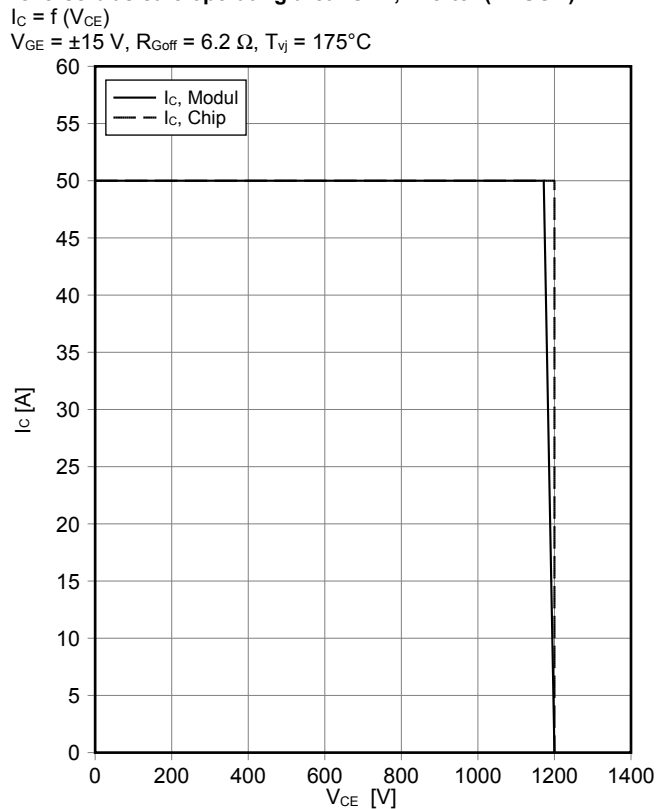
Sicherer Rückwärts-Arbeitsbereich IGBT, Wechselrichter (RBSOA) reverse bias safe operating area IGBT, Inverter (RBSOA) I_C = f(V_{CE}) V_{GE} = \pm 15\text{ V} , R_{Goff} = 6.2\ \Omega , T_{vj} = 175^\circ\text{C}
