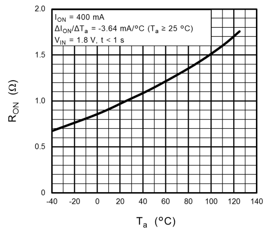
Fig. 12.4 R_{ON} - T_a
