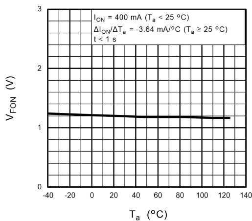
Fig. 12.5 V_{FON} - T_a
