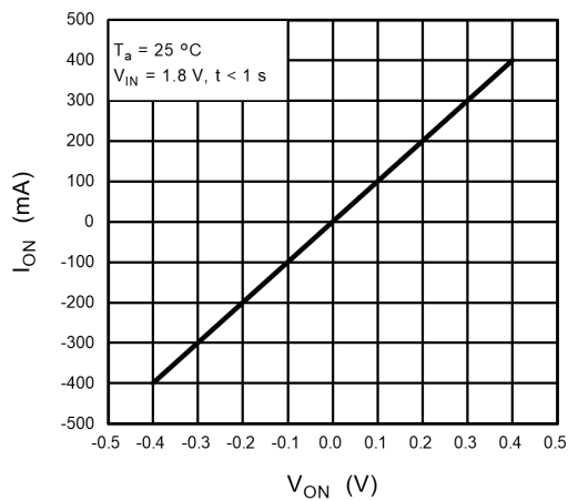
Fig. 12.3 I_{ON} - V_{ON}
