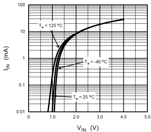
Fig. 12.1 I_{IN} - V_{IN}
