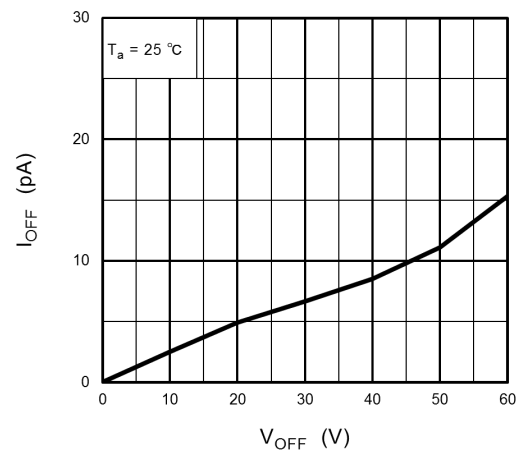
Fig. 12.8 I_{OFF} - V_{OFF}
