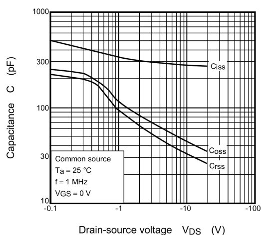
Fig. 7.9 C - V_{DS}
