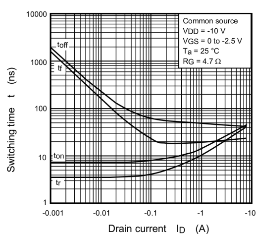
Fig. 7.10 t - I_D
