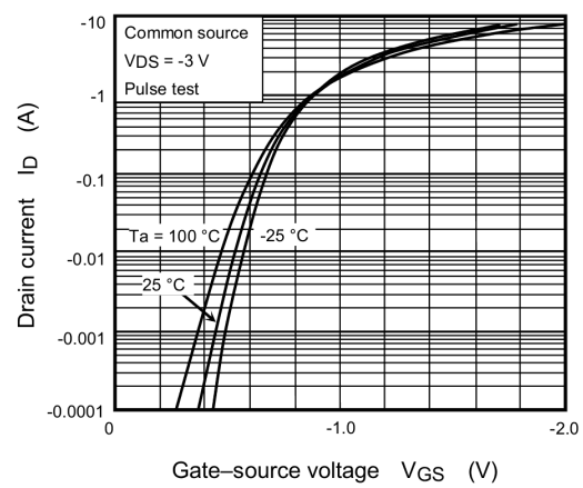
Fig. 7.2 I_D - V_{GS}
