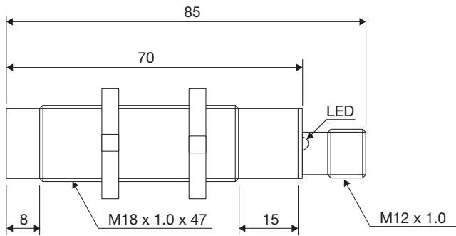
Fig. 9 Plug CA18EAN...M1IO
