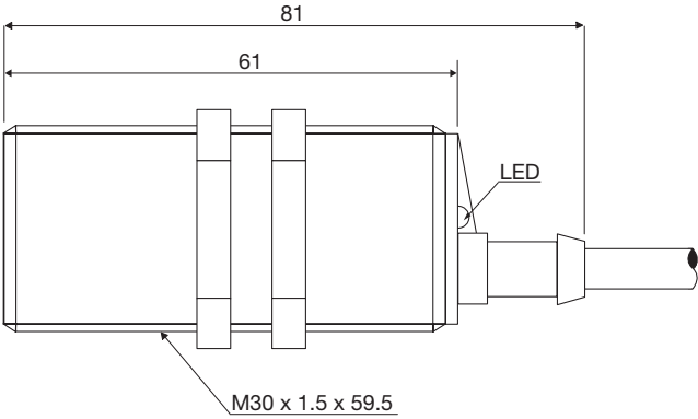
Fig. 6 Cable CA30FAF...A2IO
