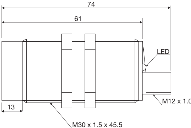
Fig. 9 Plug CA30FAN...M1IO
