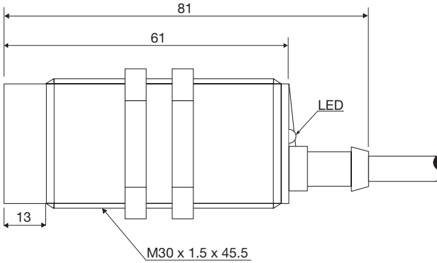
Fig. 7 Cable CA30FAN...A2IO
