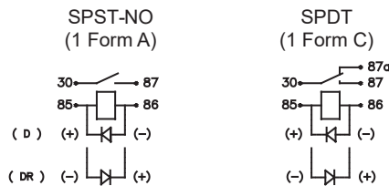
Wiring Diagrams
